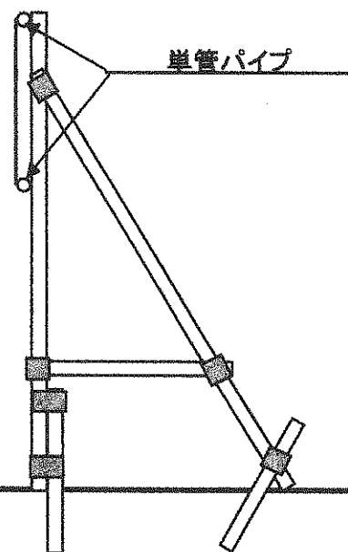
側面図
