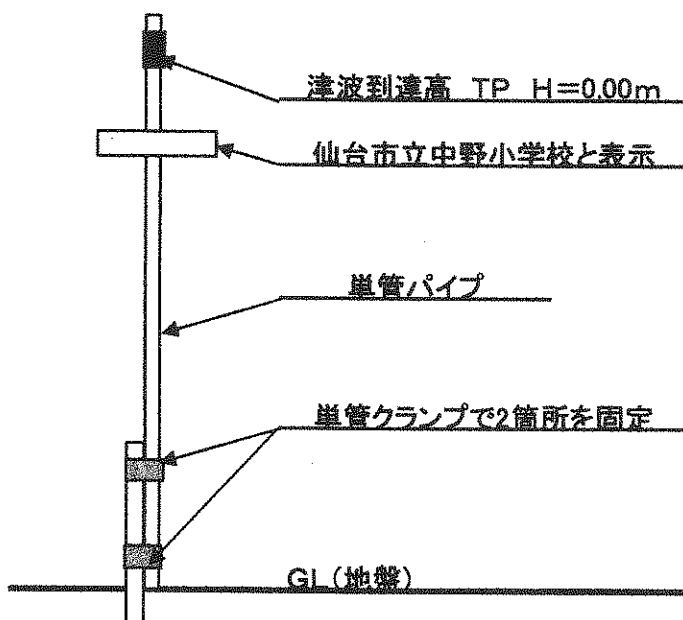
正面図
